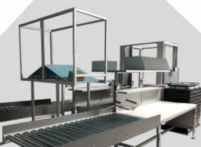
Maskinstativ och kapslingar
